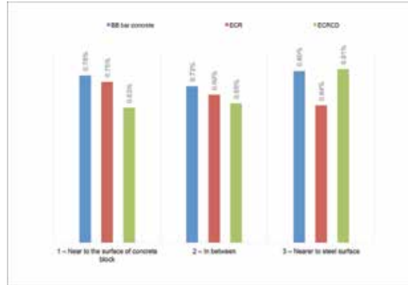
الشكل (3): تركيز الكلورايد في الكتل الخرسانية
